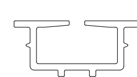
PVC CI-25 FOR 5/6mm (sku# 23-51)
