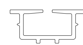
PVC CI-25 FOR 5/6mm (sku# 23-51)
