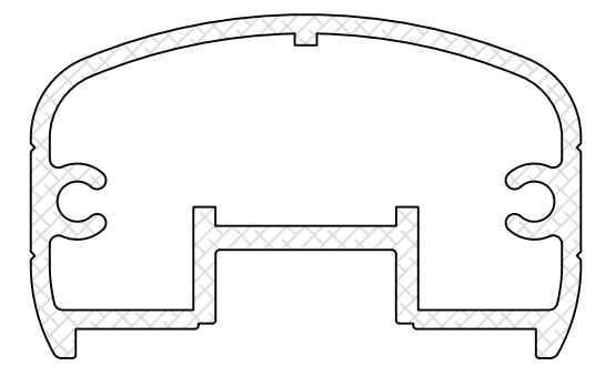
1250 TOP RAIL (sku# 50-30)
