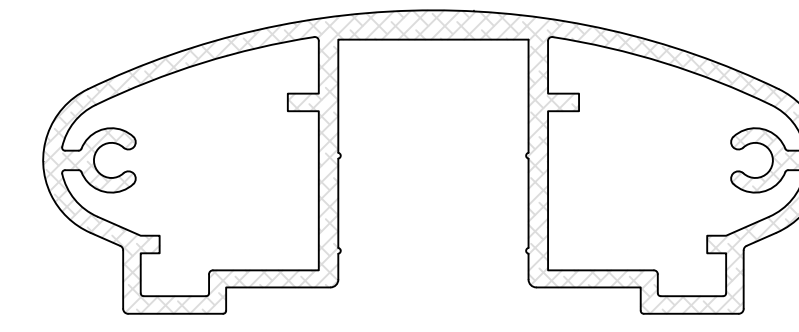
6000R TOP RAIL (sku# 60-220)
