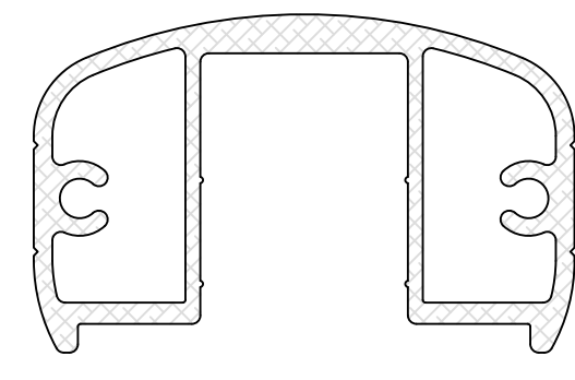
1255 TOP RAIL (sku# 50-35)
