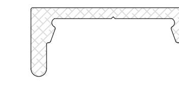
HD-WP BOTTOM RAIL (sku# 74-40)
