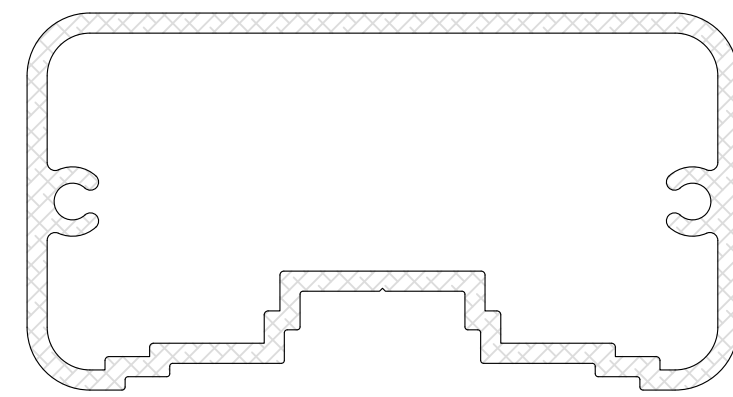
3500S TOP RAIL (sku# 30-35)
