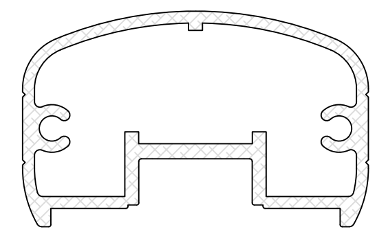
1250 TOP RAIL (sku# 50-30)
