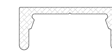
HD-WP BOTTOM RAIL (sku# 74-40)
