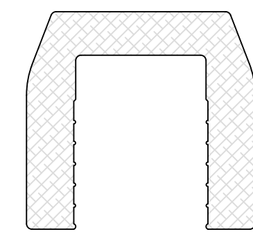
2200 MID RAIL (sku# 22-05)
