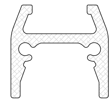
2200 BOTTOM RAIL (sku# 22-02)
