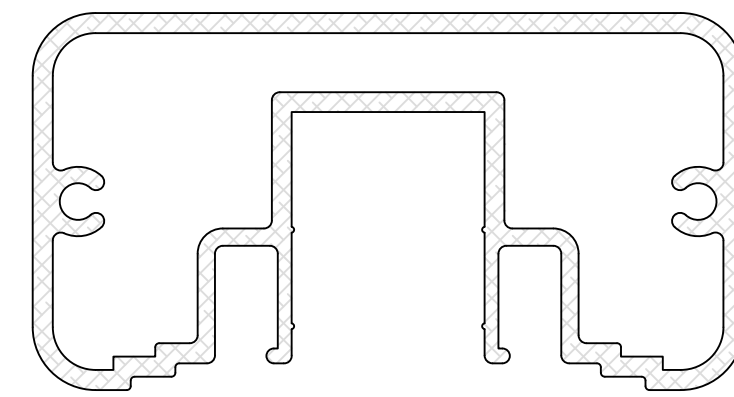
3600S TOP RAIL (sku# 30-36)
