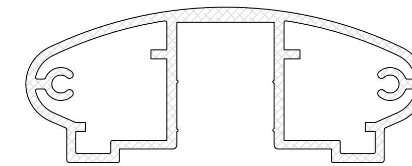
6000R TOP RAIL (sku# 60-220)
